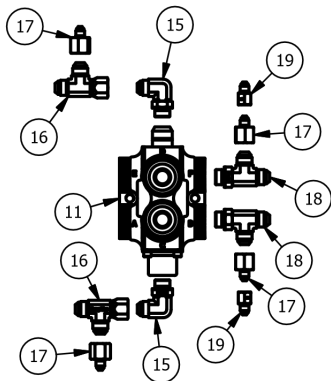
2WD/4WD VALVE (SD40)
