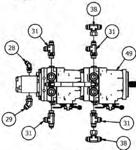
HYDROSTAT
