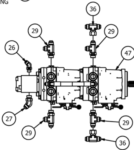
HYDROSTAT
