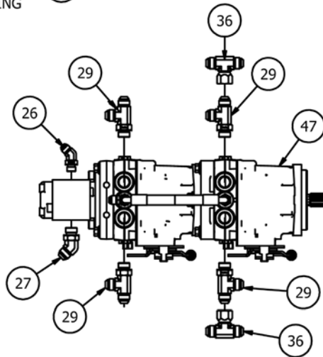
HYDROSTAT
