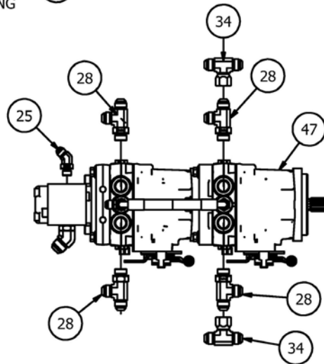
HYDROSTAT
