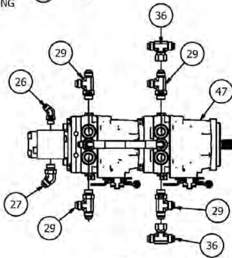
HYDROSTAT
