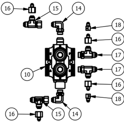
2WD/4WD VALVE (SD40)
