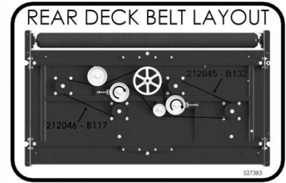
ITEM 15 527383
