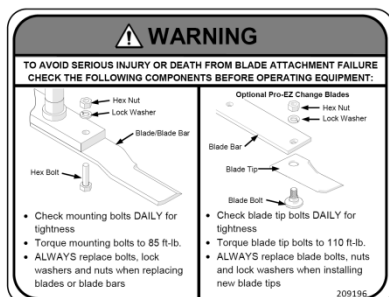
ITEM 19 (209196)
