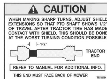
ITEM 2 (209171)
