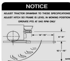
ITEM 10 (521784)
