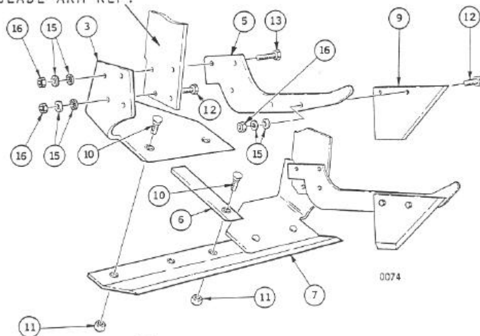
1 3 PIECE UNIBLADE, 16"
